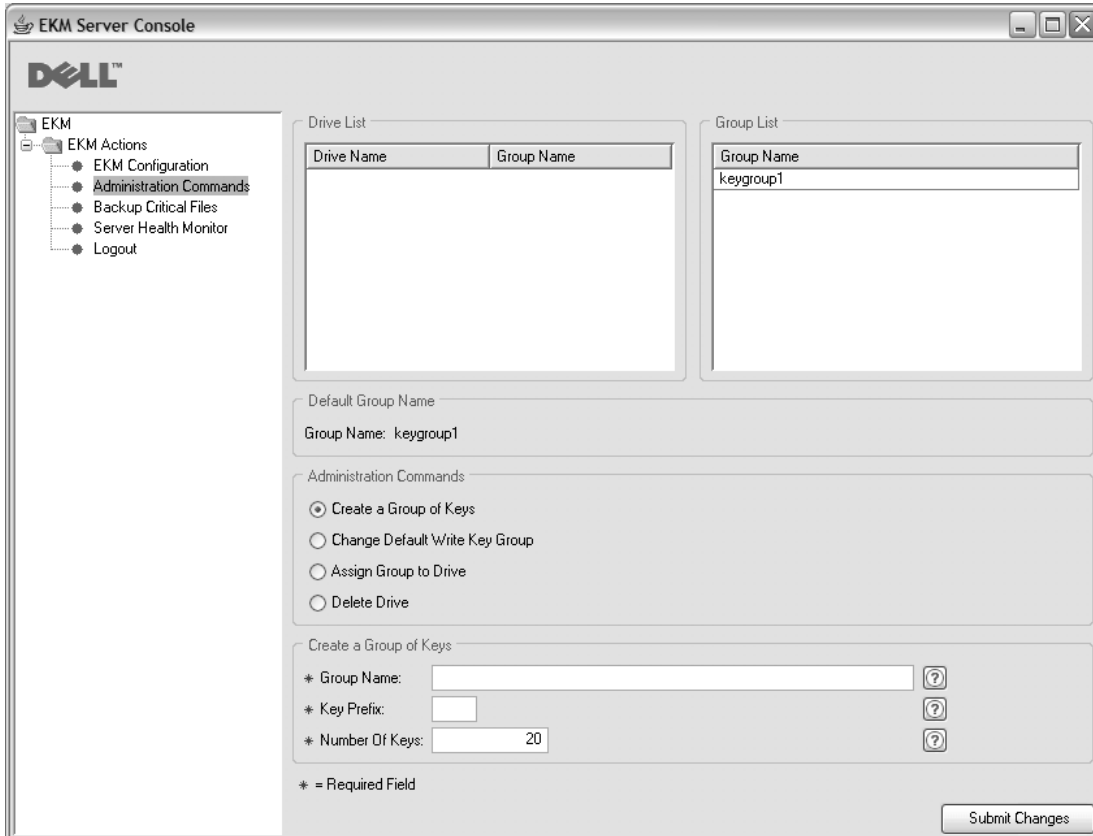
图 3-7. 创建密钥组
